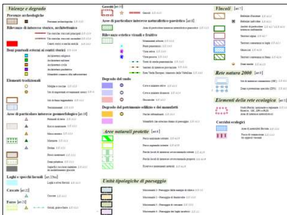
Figura n° 12 - Estratto PTCP Provincia di Sondrio Tavola 4.06 – “Elementi Paesistici e Rete ecologica”. Area oggetto di intervento evidenziata dal cerchio rosso.
