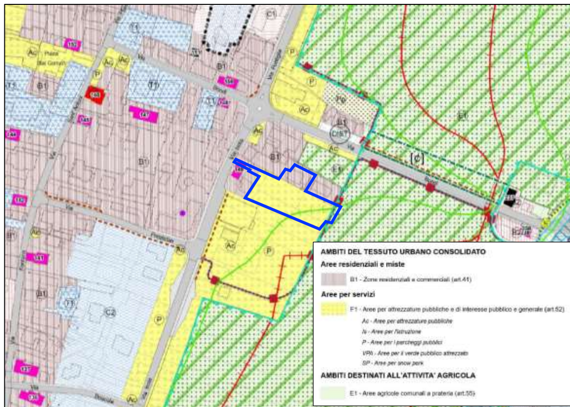
Figura n° 7 - Estratto Tav. 7.2 Var Piano delle Regole P.G.T. di Livigno.
