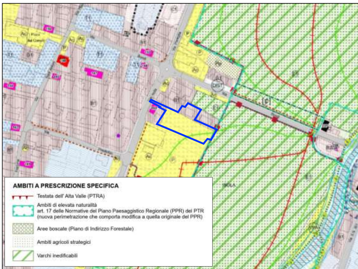
Figura n° 10 - Estratto Tav. 7.2_TessutoUrbanoConsolidato_2000_6VAR del PDR del P.G.T. del vigente del Comune di Livigno. Area oggetto di intervento evidenziata dal poligono blu.
