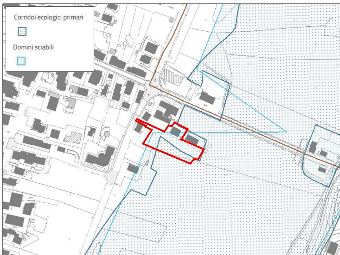
Figura n° 13 – Estratto cartografia “PTRA Media e Alta Valtellina” (fonte Geoportale Regione Lombardia). Area oggetto di intervento evidenziata dal poligono rosso.
