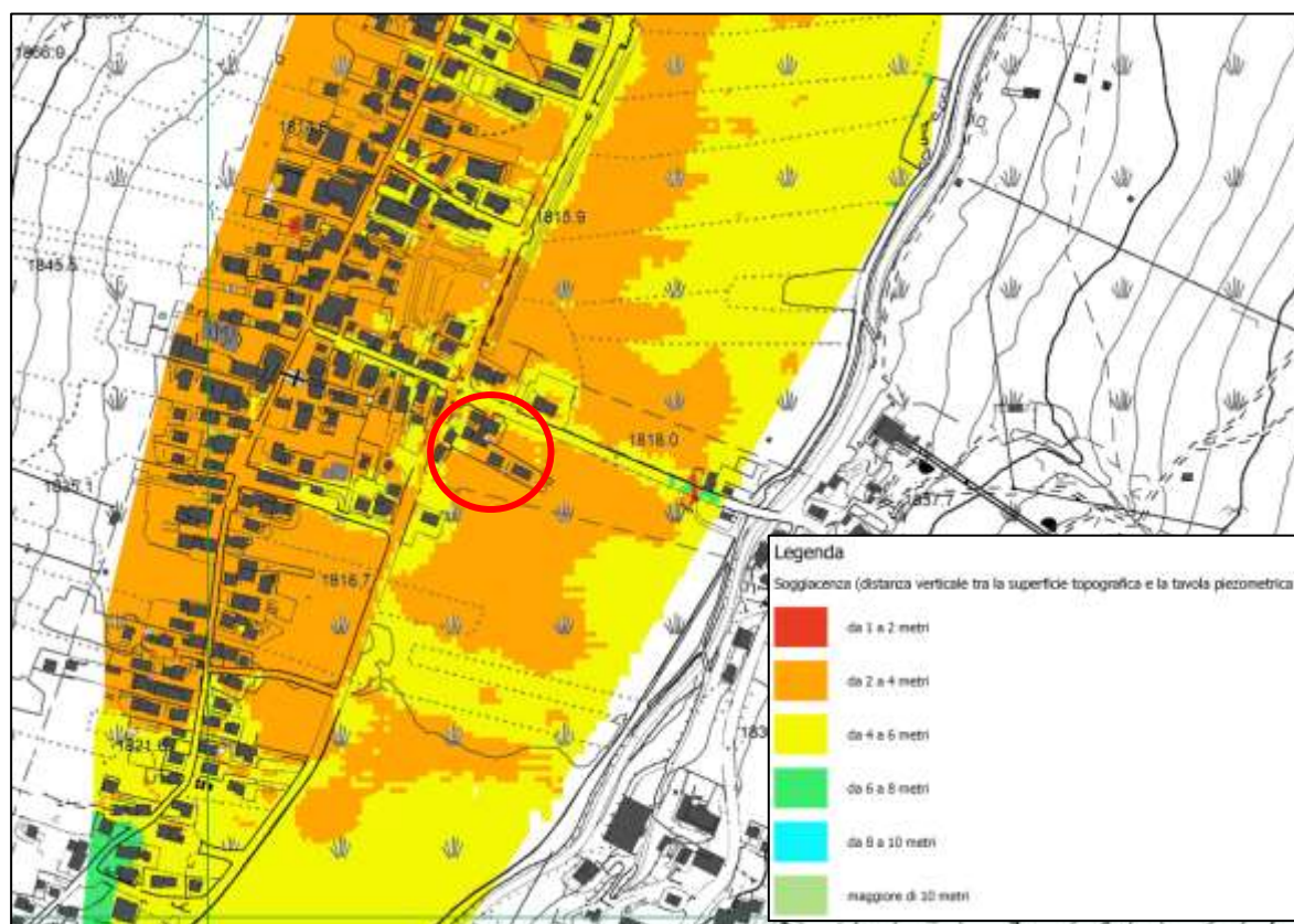
Figura n° 6 – Stralcio “Carta della soggiacenza” del PGT di Livigno
