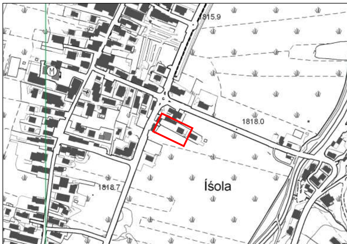
Figura n° 1 - Estratto CTR Sez. D1a4 Area oggetto del P.I.I. evidenziata dal rettangolo rosso
