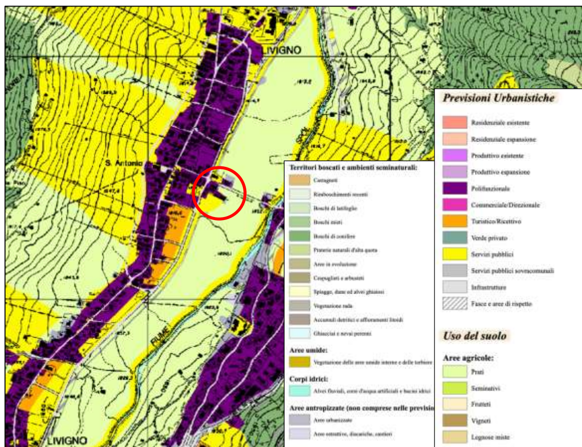
Figura n° 11 - Estratto PTCP Provincia di Sondrio Tavola 2.06 – “Uso del suolo e Previsioni urbanistiche”. Area oggetto di intervento evidenziata dal cerchio rosso.
