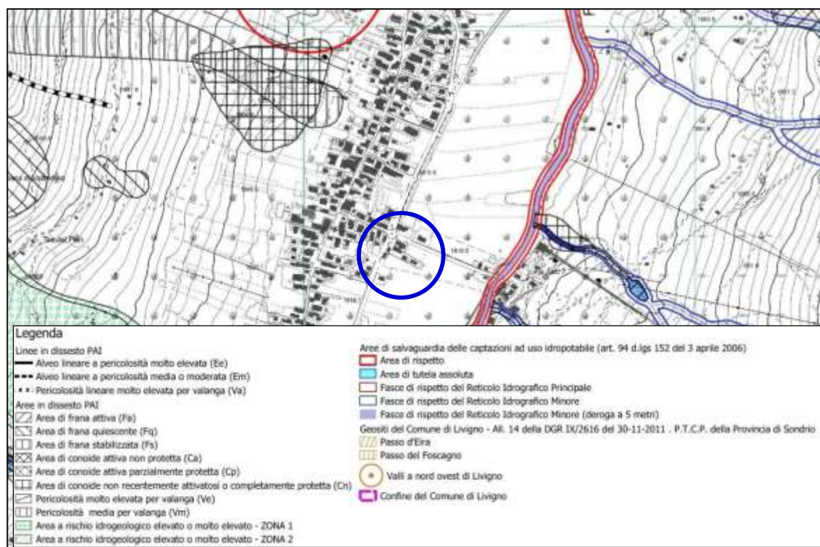
Figura n° 16 - Estratto Carta dei vincoli" del P.G.T. del Comune di Livigno Area di intervento evidenziata dal cerchio blu.
