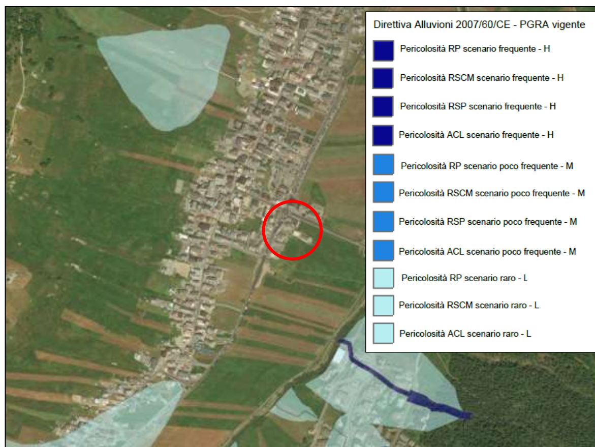
Figura n° 18 - Estratto carta Direttiva Alluvioni 2007/60/CE – PGRA Vigente 28/11/2025 - Pericolosità (fonte Geoportale Regione Lombardia). Area di intervento evidenziata dal cerchio rosso.
