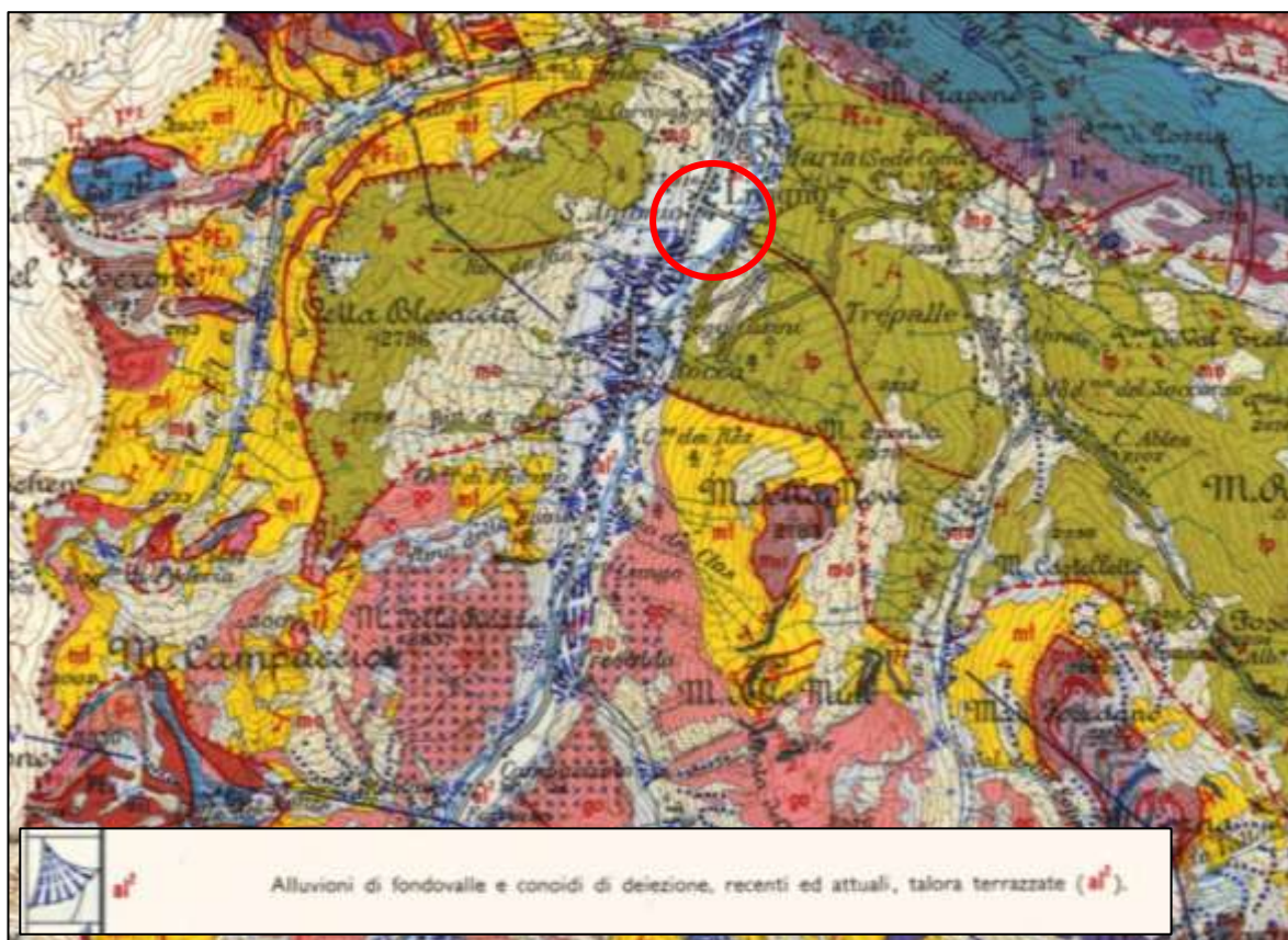
Figura n° 5 – Carta geologica d'Italia 1 : 100.000 "Foglio 8 Bormio" e relativa legenda
