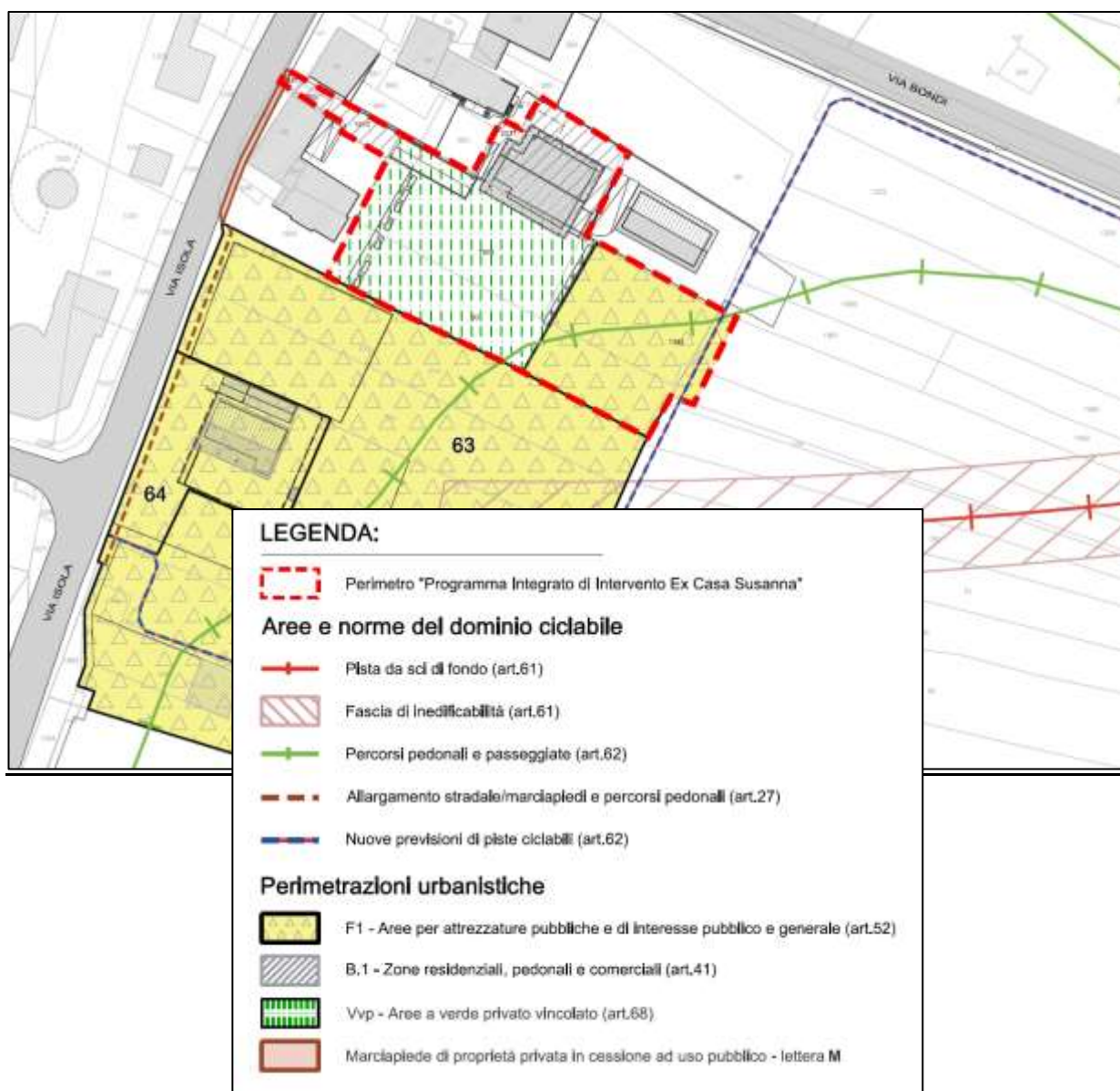
Figura n° 8 - Stralcio elaborato progettuale estratto dalla "TAV- N°2 – ALLEGATO N°1 – INQUADRAMENTO URBANISTICO - VARIANTE -PLANIMETRIA GENERALE"
