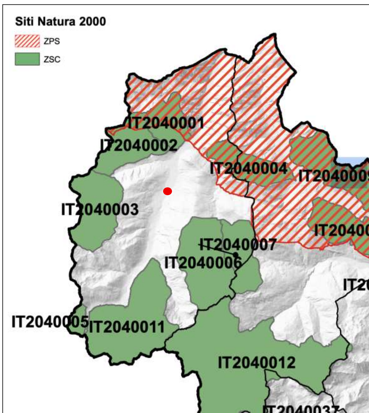
Figura n° 19 - Estratto Cartina di Inquadratura Siti Natura 2000 (fonte Provincia di Sondrio). Area di intervento evidenziata dal cerchio rosso.
